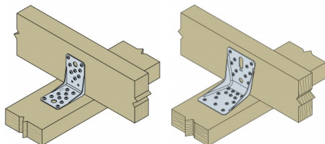
Fijación madera/soporte rígido
