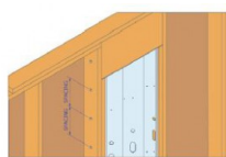
Etapa 3 : Unalas con los montantes adyacentes
