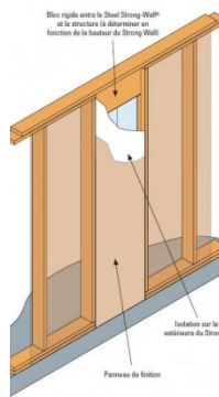
Etapa 4 : Instale un bloque rígido entre el muro
